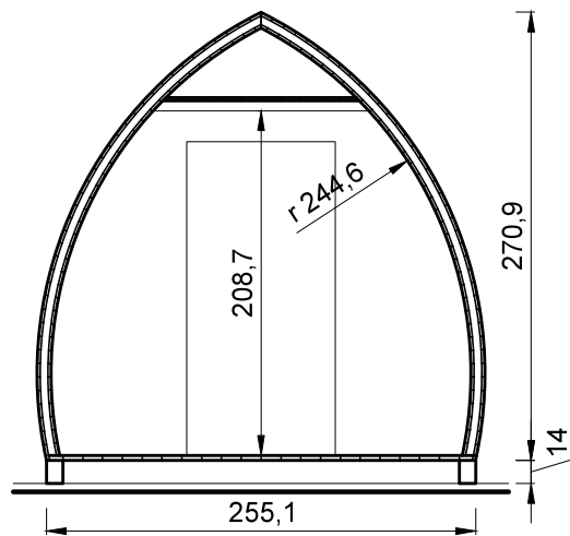
SEZIONE
