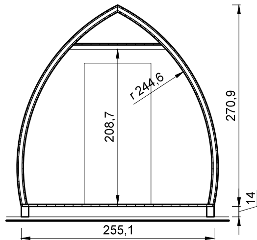
SEZIONE
